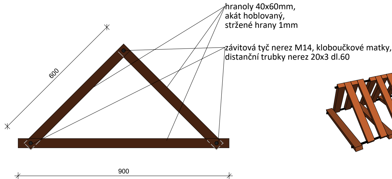
POHLED BOČNÍ
