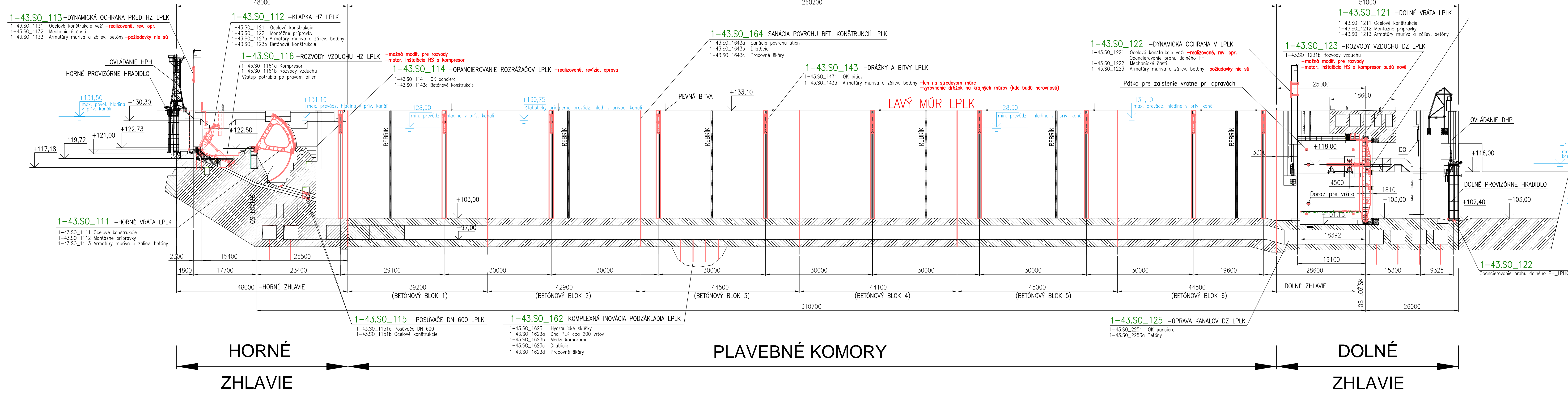
A-A POZDLŽNY REZ LPLK 1-43.SO_1
