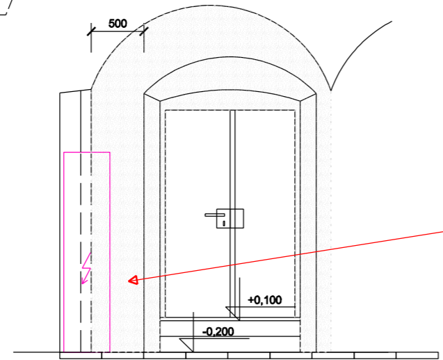
Řez H - H
