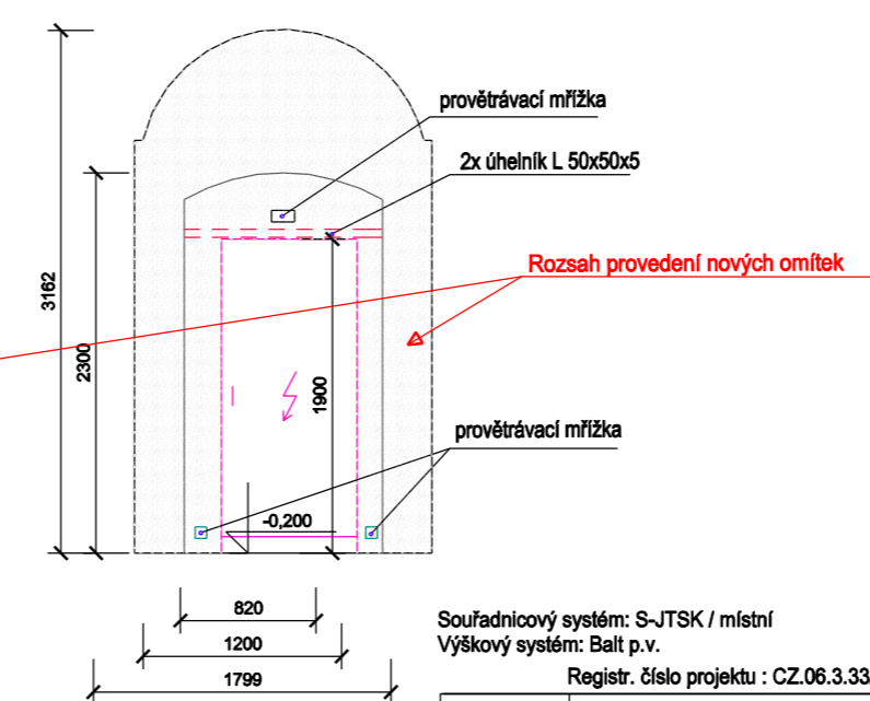
Řez F - F
