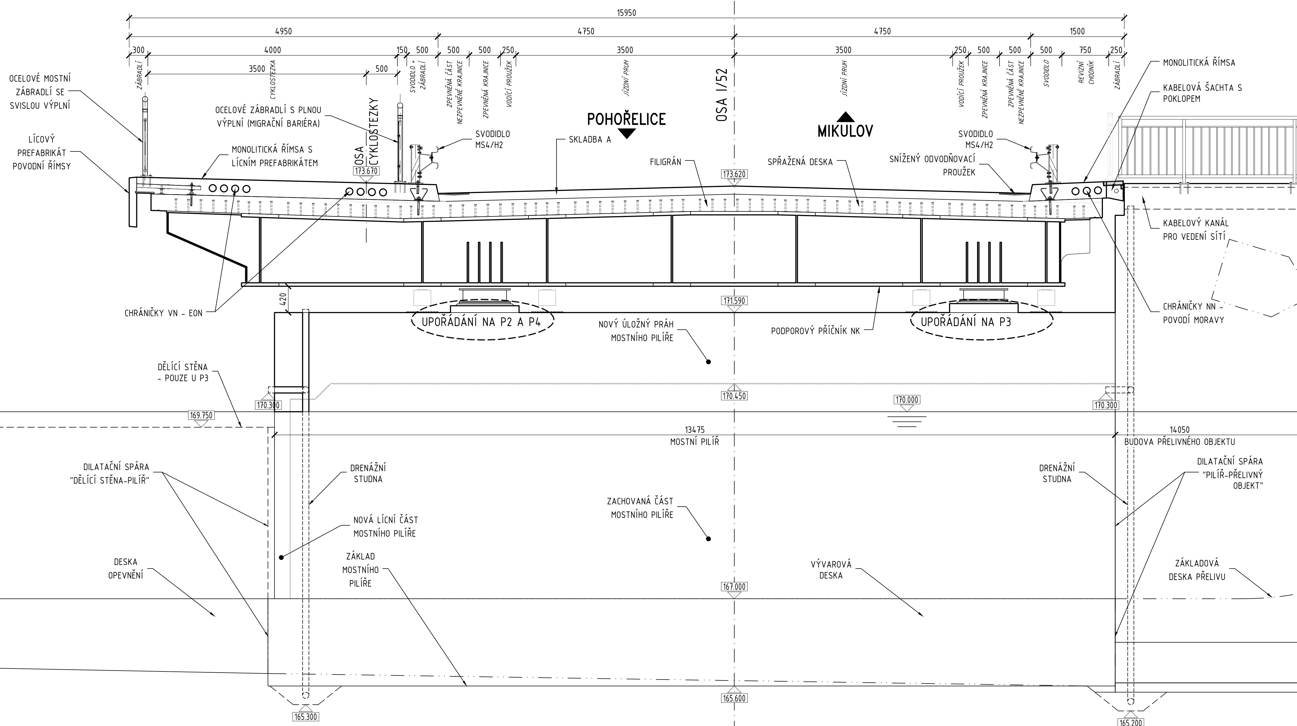
PŘÍČNÝ ŘEZ OSOU ULOŽENÍ NA PILÍŘÍCH 1:35
