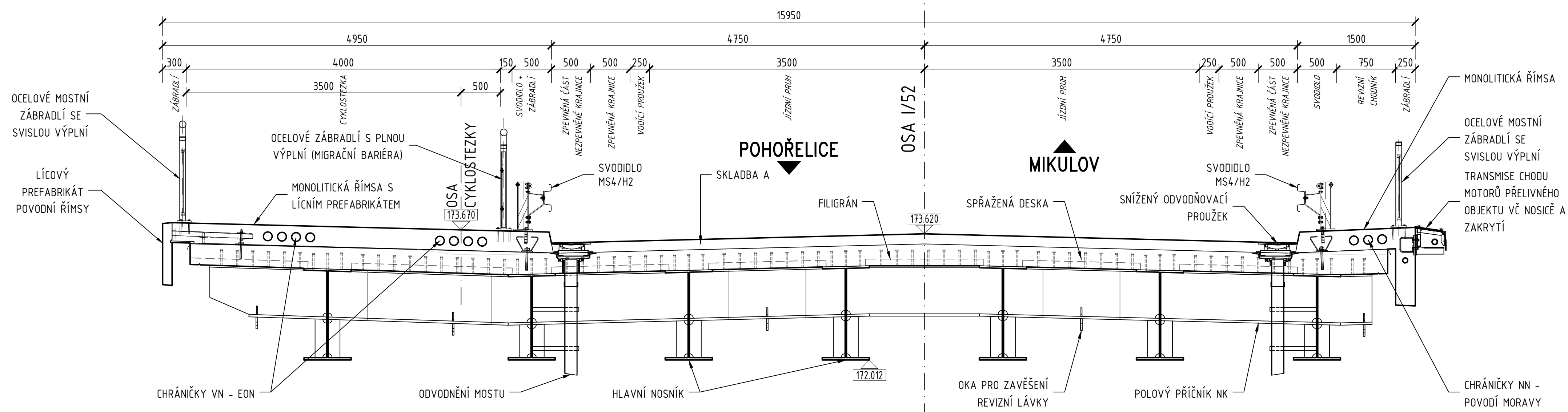
PŘÍČNÝ ŘEZ VE VNITŘNÍCH POLÍCH 1:35
