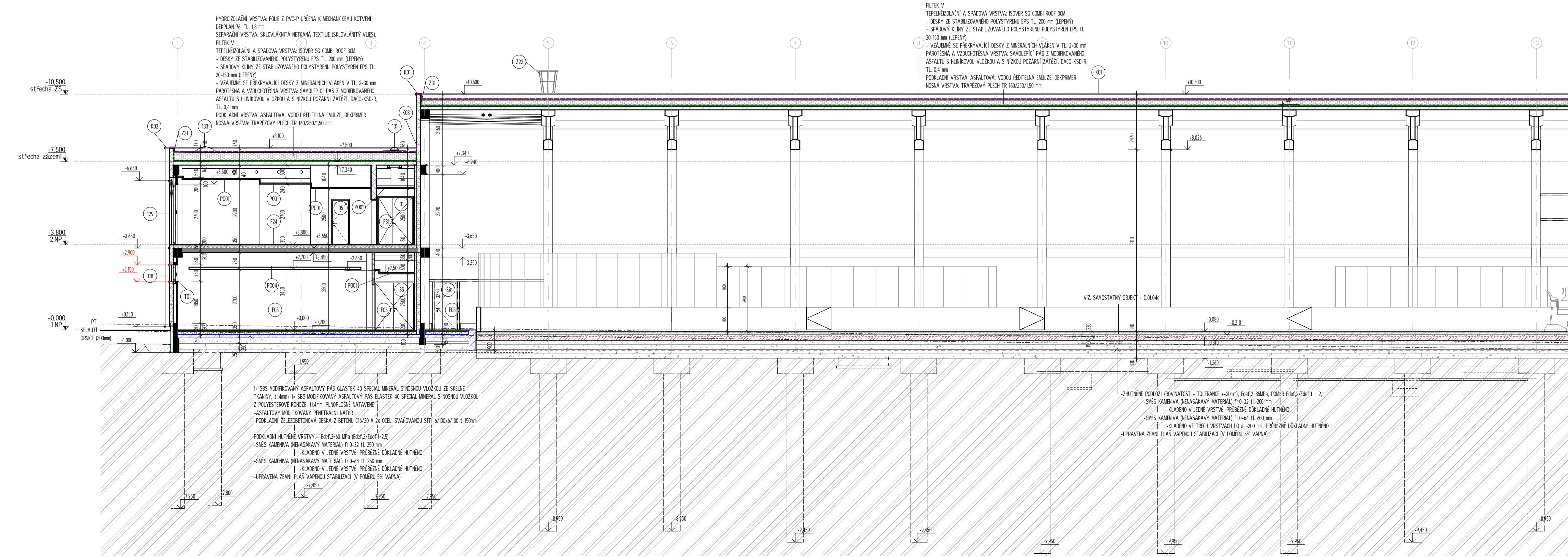
Řez B-B'
